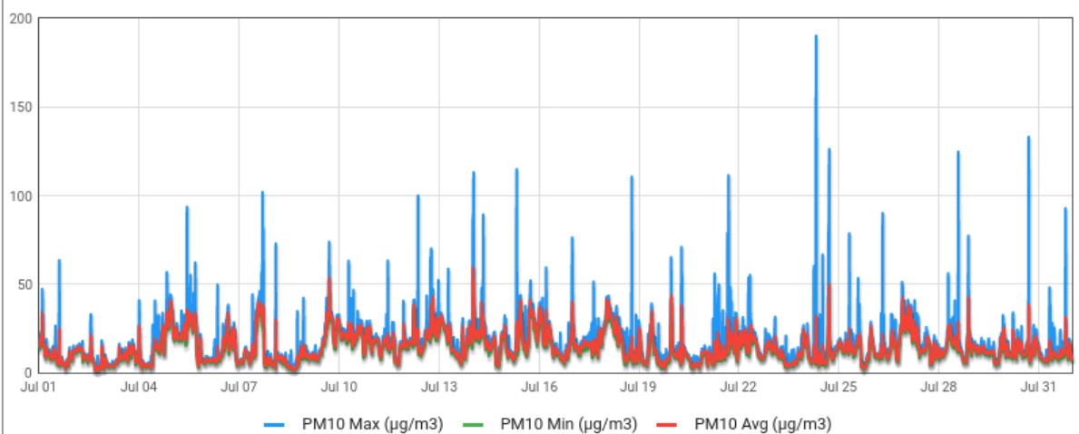
Concentración de masa: Material particulado PM10
