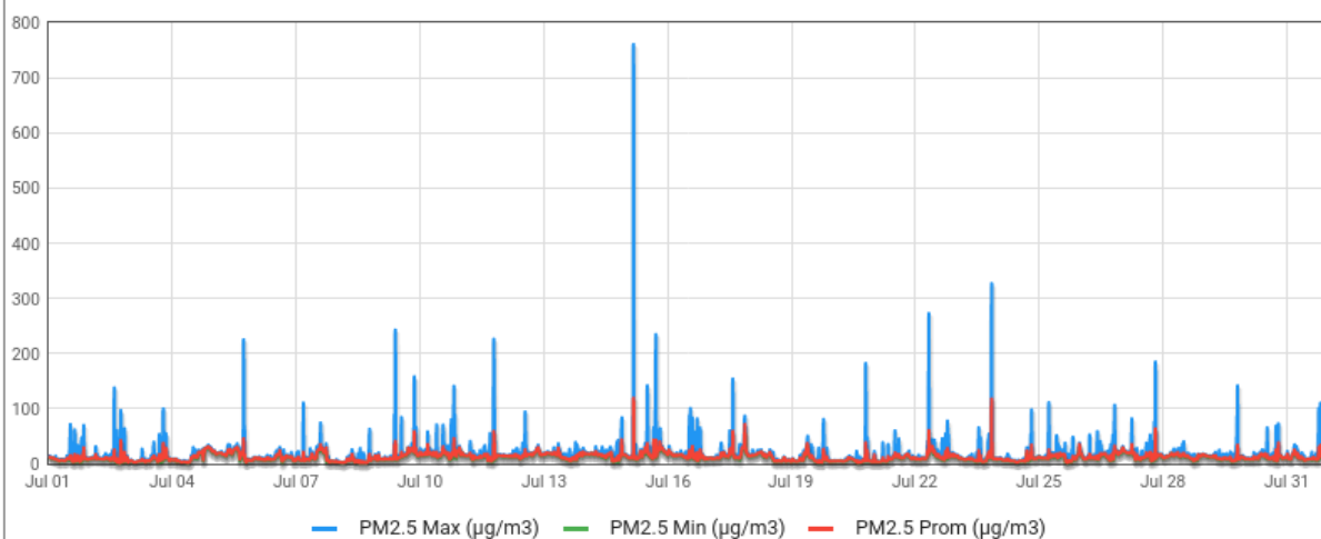
Concentración de masa: Material particulado PM2.5
